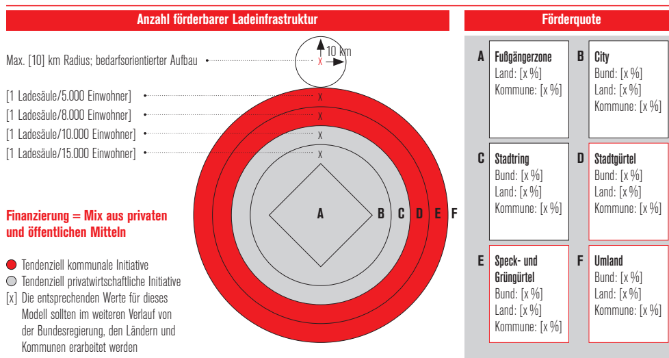
Abbildung 15: Systematik des Modells SIMONE
